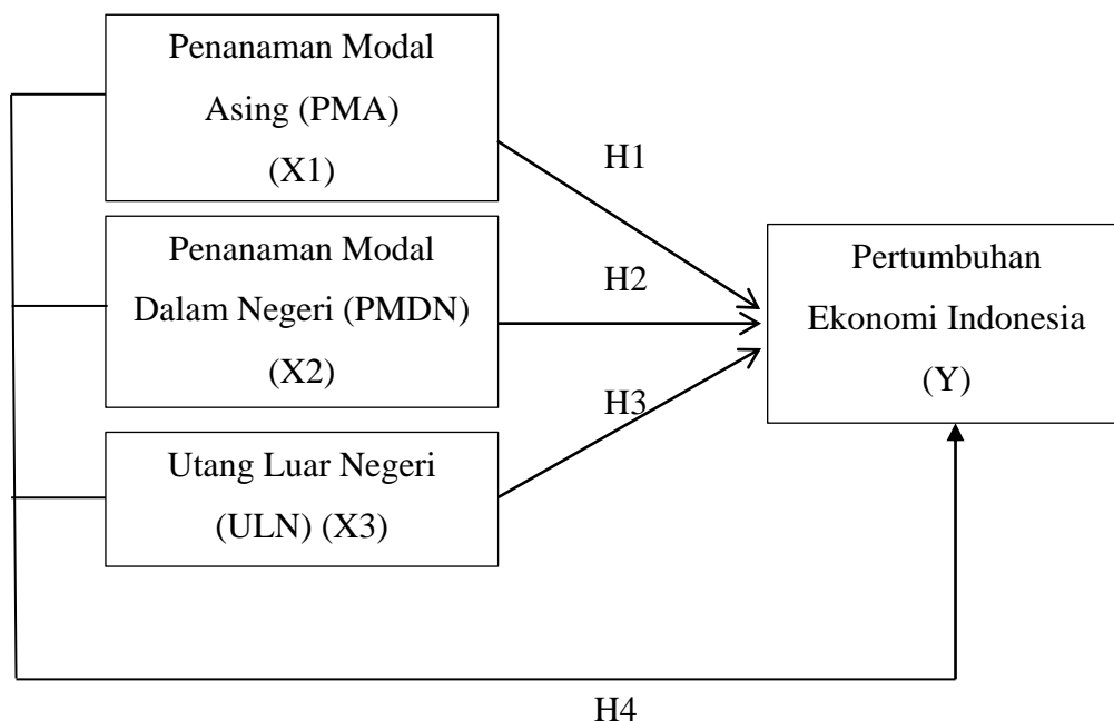
Gambar 2. 1 Kerangka Berpikir
