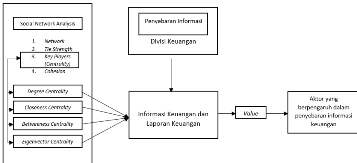
Gambar 1 Kerangka Pemikiran
